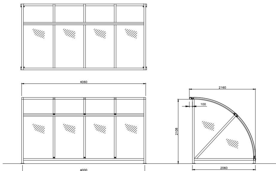
Figure 3. Dimensions de l'abri vélos
